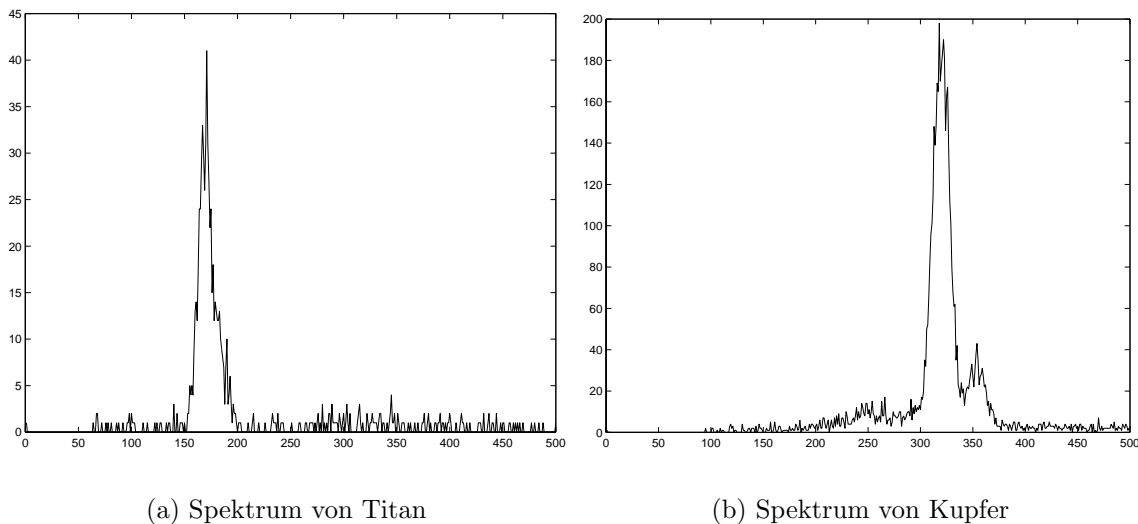
Abbildung 3.8: Spektren, die durch Erstellen eines Histogramms unter Berücksichtigung der Mehrpixelereignisse aus den CCD-Aufnahmen gewonnen wurden. Mit der Summationsmethode werden nur Signale oberhalb eines eingestellten Schwellwertes erfaßt.
