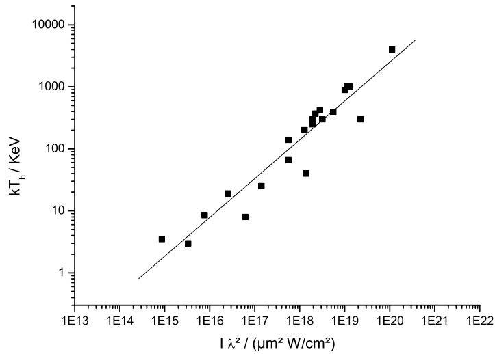
Abbildung 2.1: Abhängigkeit der heißen Elektronentemperatur von I \lambda^2 nach [12].
